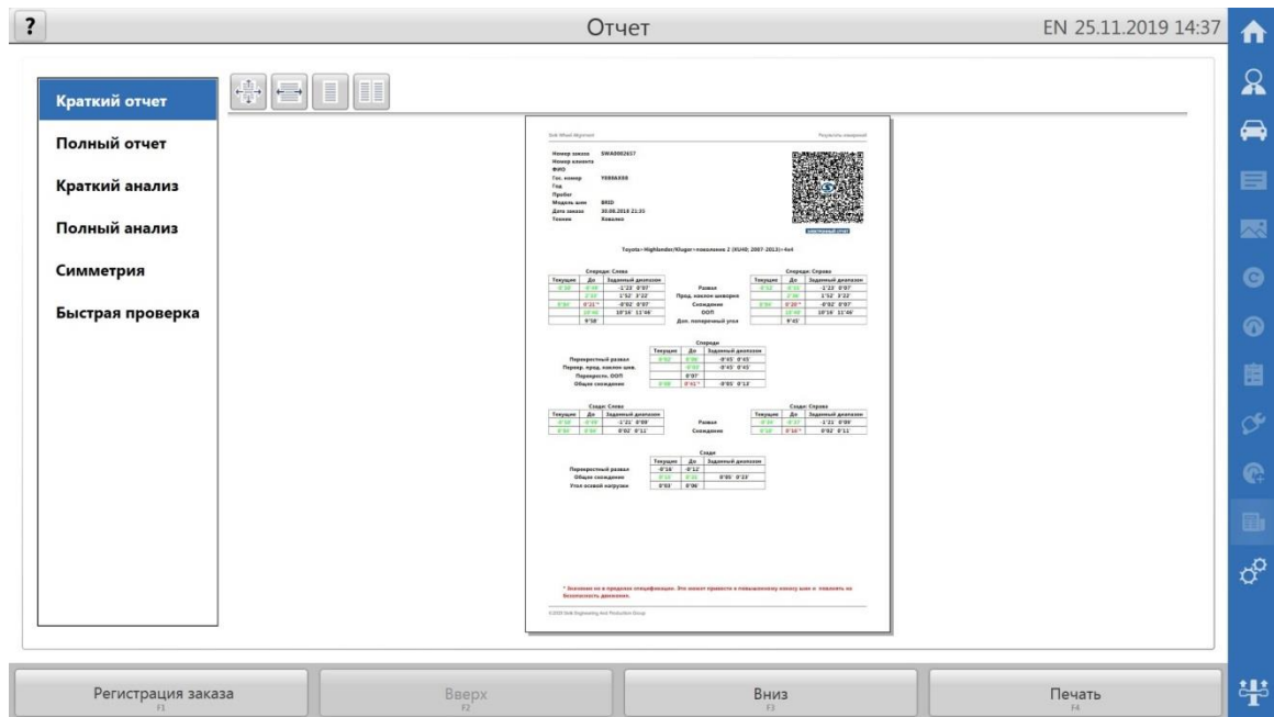
Рисунок 6.29 - Окно отчетов
